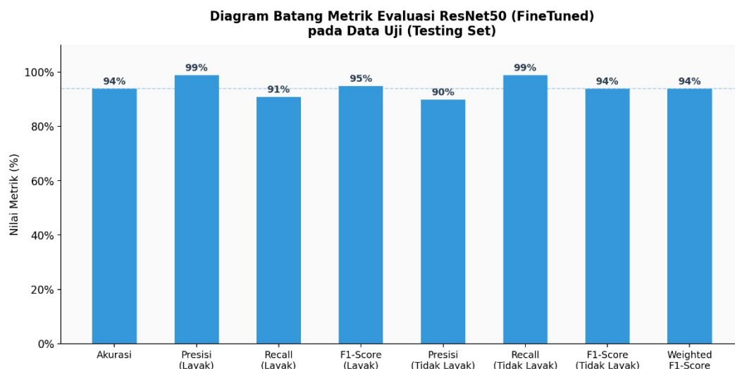
Gambar 4.7 Diagram Batang Metrik Evaluasi ResNet50 (Fine-Tuned) pada Data Uji
