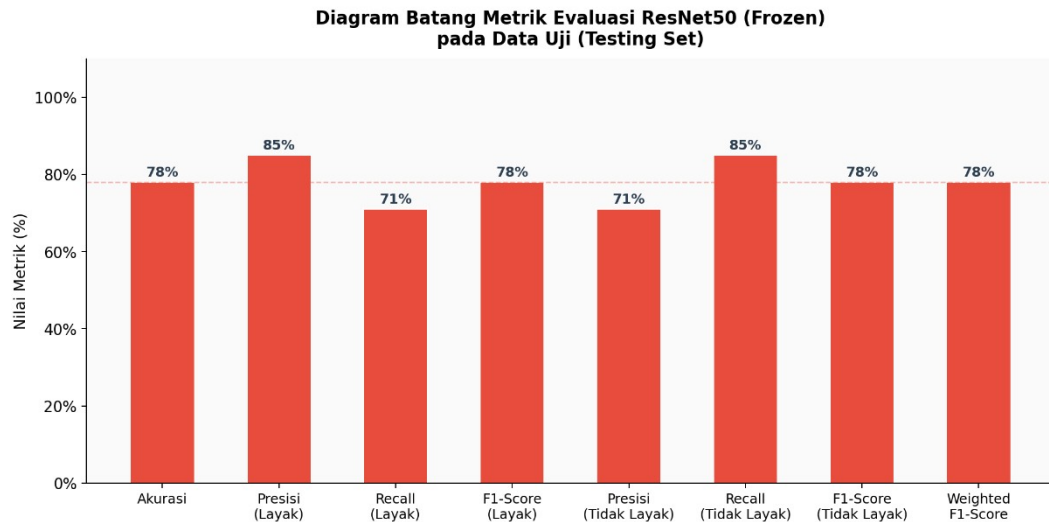
Gambar 4.5 Diagram Batang Metrik Evaluasi ResNet50 (Frozen) pada Data Uji
