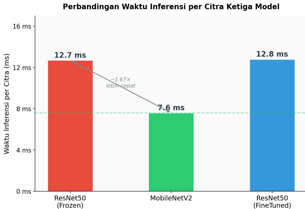
Gambar 4.12 Diagram Batang Perbandingan Waktu Inferensi per Citra Ketiga Model
