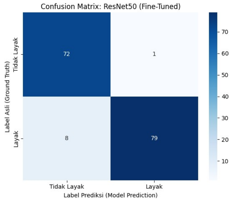
Gambar 4.10 Confusion Matrix ResNet50 Fine-Tuned pada Data Uji
