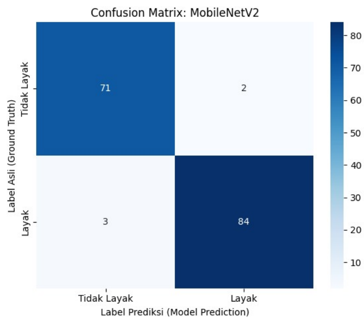
Gambar 4.9 Confusion Matrix MobileNetV2 pada Data Uji
