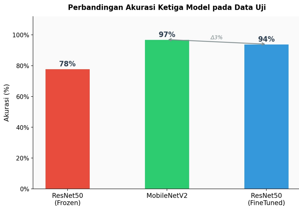
Gambar 4.11 Diagram Batang Perbandingan Akurasi Ketiga Model pada Data Uji
