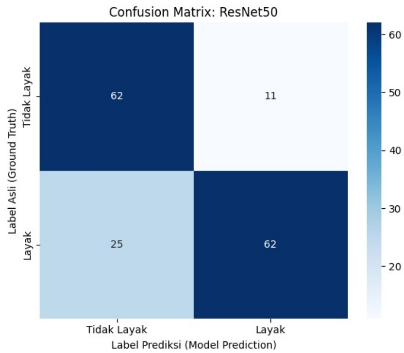
Gambar 4.8 Confusion Matrix ResNet50 pada Data Uji
