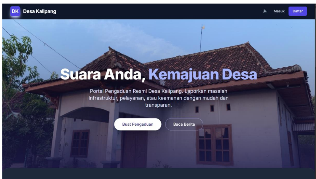
Gambar 4. 6 Halaman Beranda
